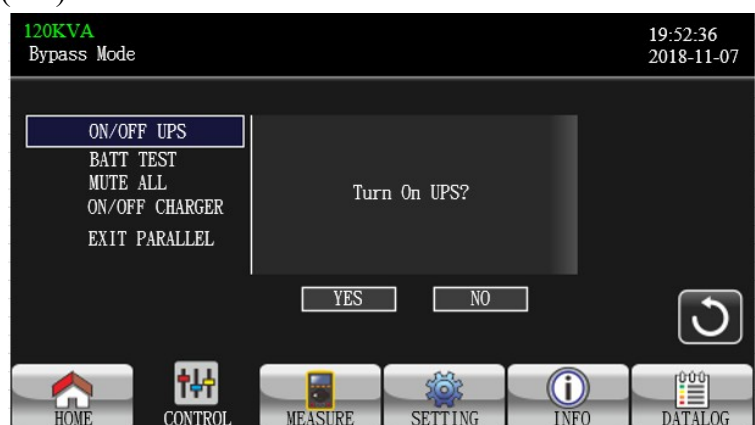
Рисунок 12. Подтверждение включения
