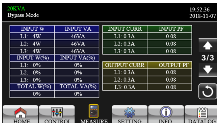
Рисунок 15. Страница 3 меню «Измерения»
