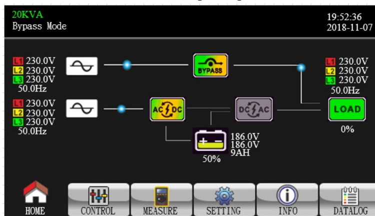
Рисунок 9. Основной экран ИБП
