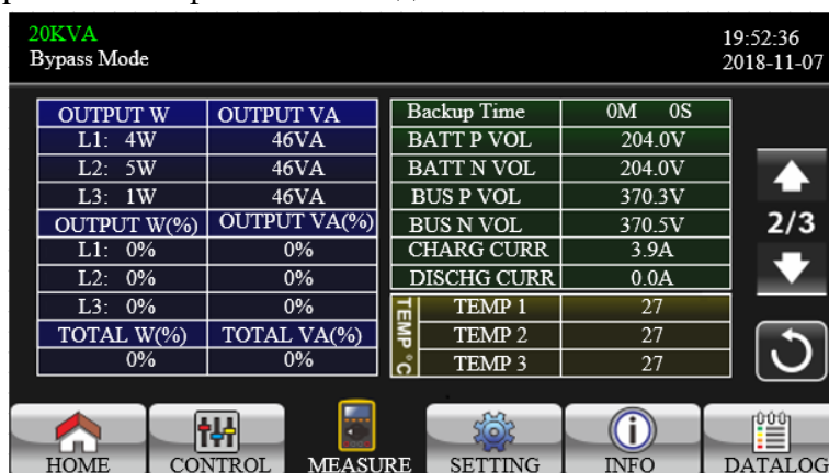
Рисунок 14. Страница 2 меню «Измерения»
