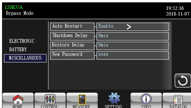
Рисунок 21. Подменю MISCELLANEOUS
