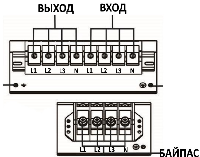
Рисунок 5. Блок клемм XF60
