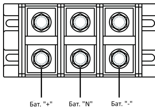
Рисунок 5. Блок клемм XF60
