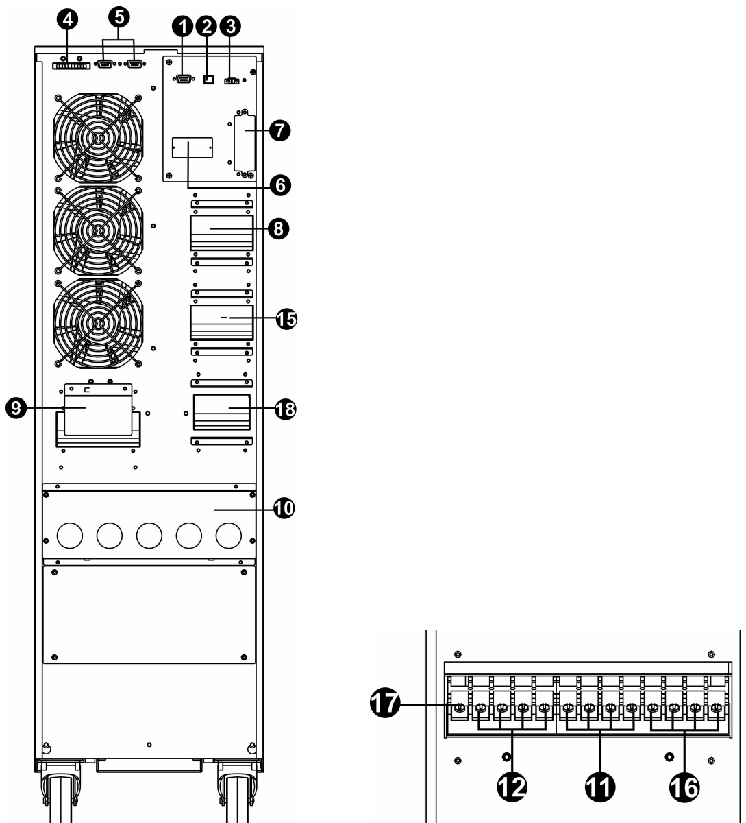
Рисунок 1. Задняя панель и клеммы подключения XF40
