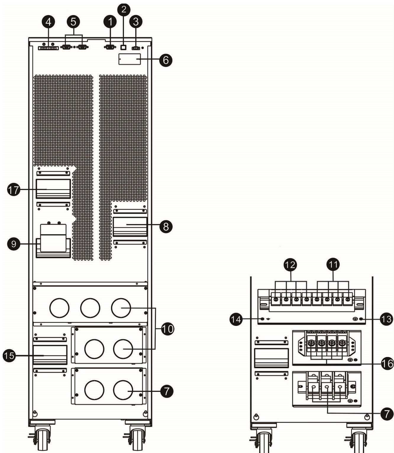
Рисунок 2. Задняя панель и клеммы подключения XF60
