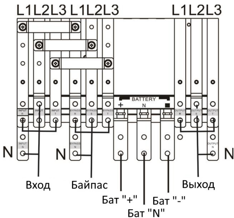
Рисунок 7. Блок клемм XF100/120/180/200
