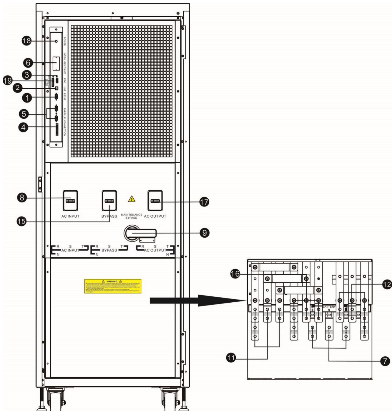
Рисунок 4. Передняя панель(дверь открыта) и клеммы подключения XF180/200
