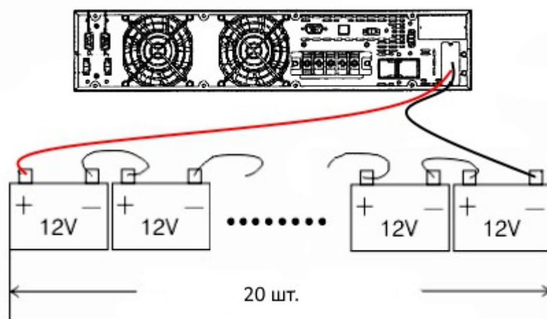
Схема подключения комплекта внешних АКБ.
