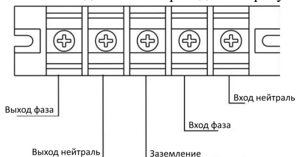
Рис.2 Подключение ИБП
