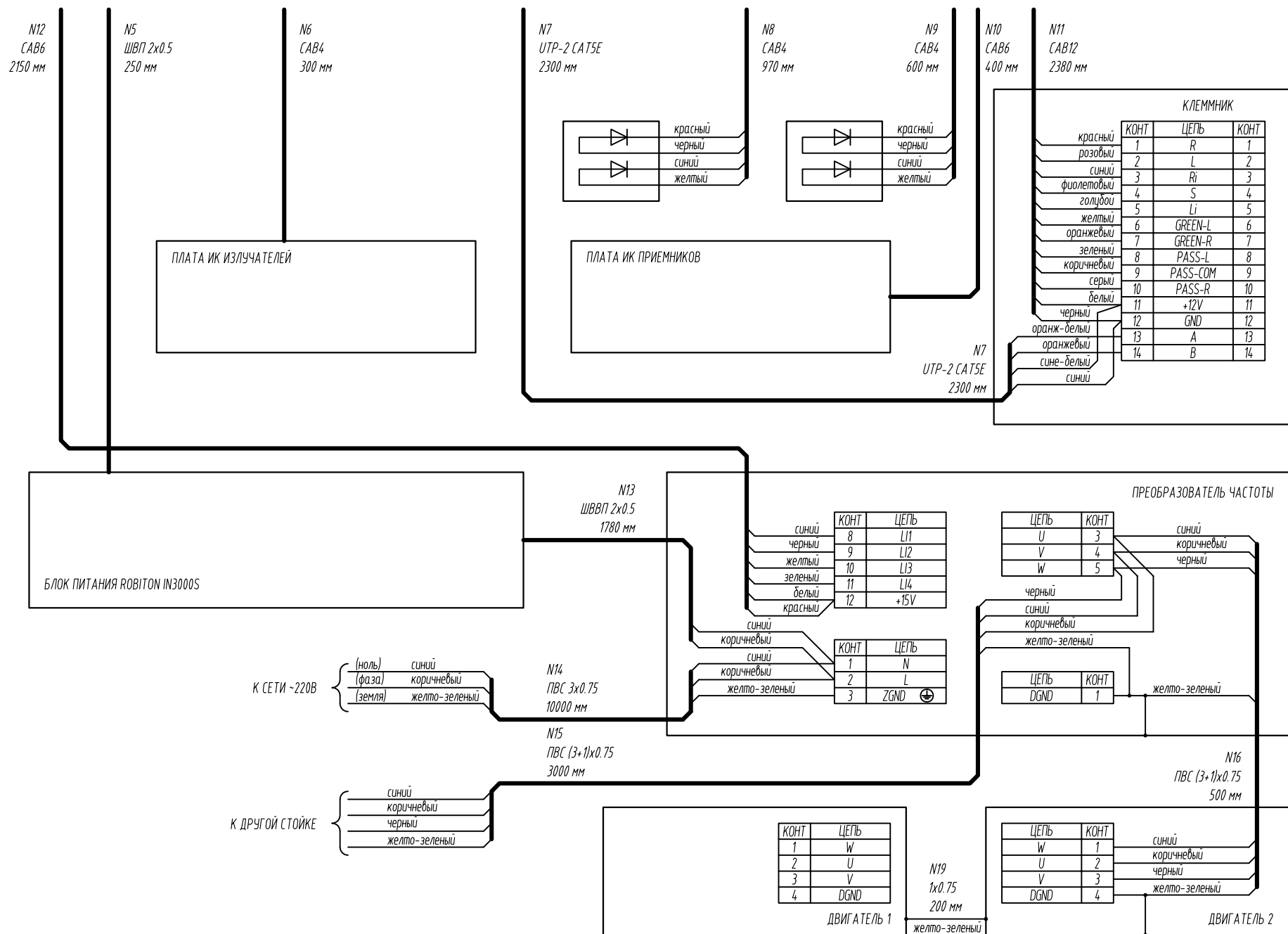
Схема внутristоечных соединений МАТ-ОМА-Ш дуплекс ОМА-86.68х_5 лист 2 из 2
