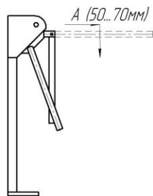
Рис.2 Штанга-антипаника
