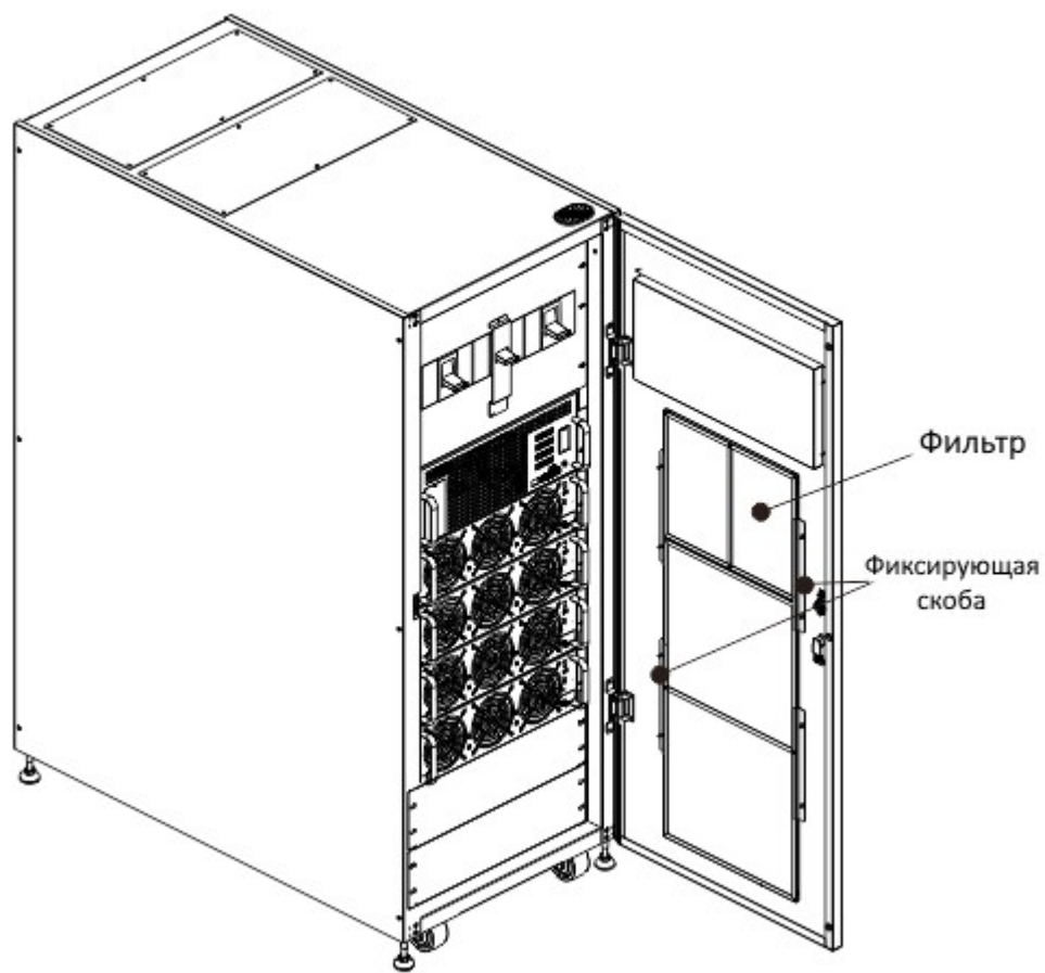
Рисунок 28. Фильтрующие элементы.
