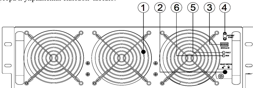
Рисунок 12. Силовой модуль.
