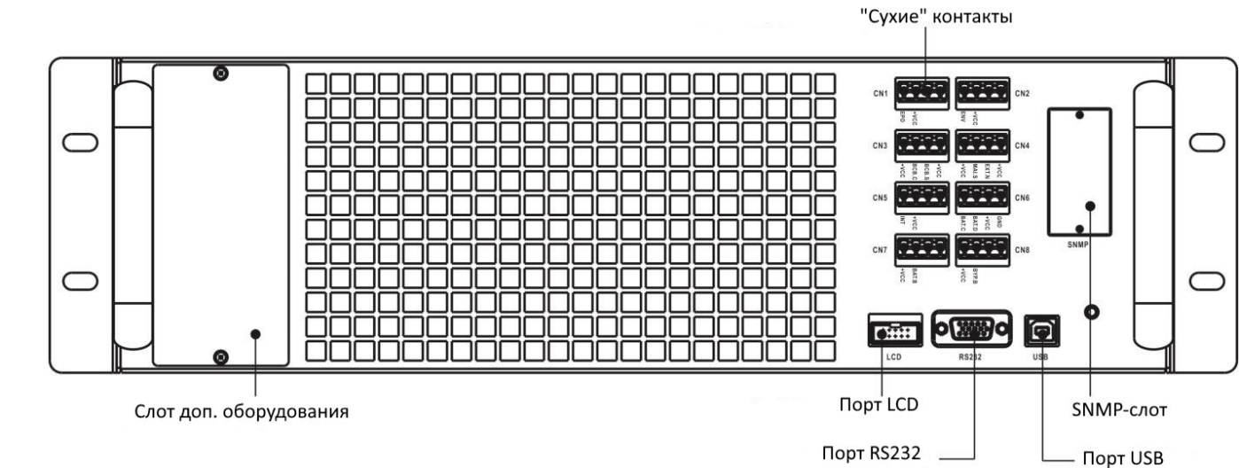
Рисунок 27. Коммуникационные интерфейсы.
