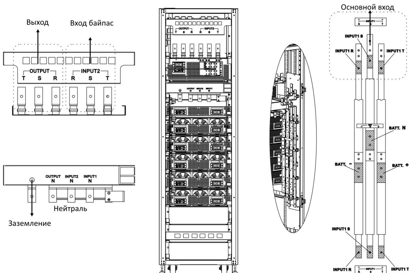
Рисунок 8. Шины подключения XM4 300.
