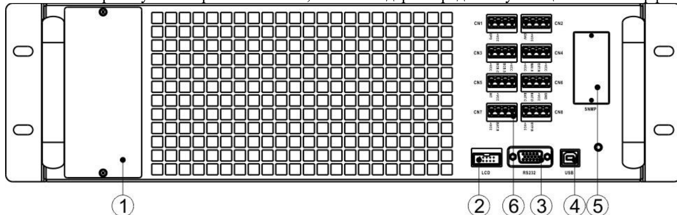
Рисунок 11. Модуль байпаса.
