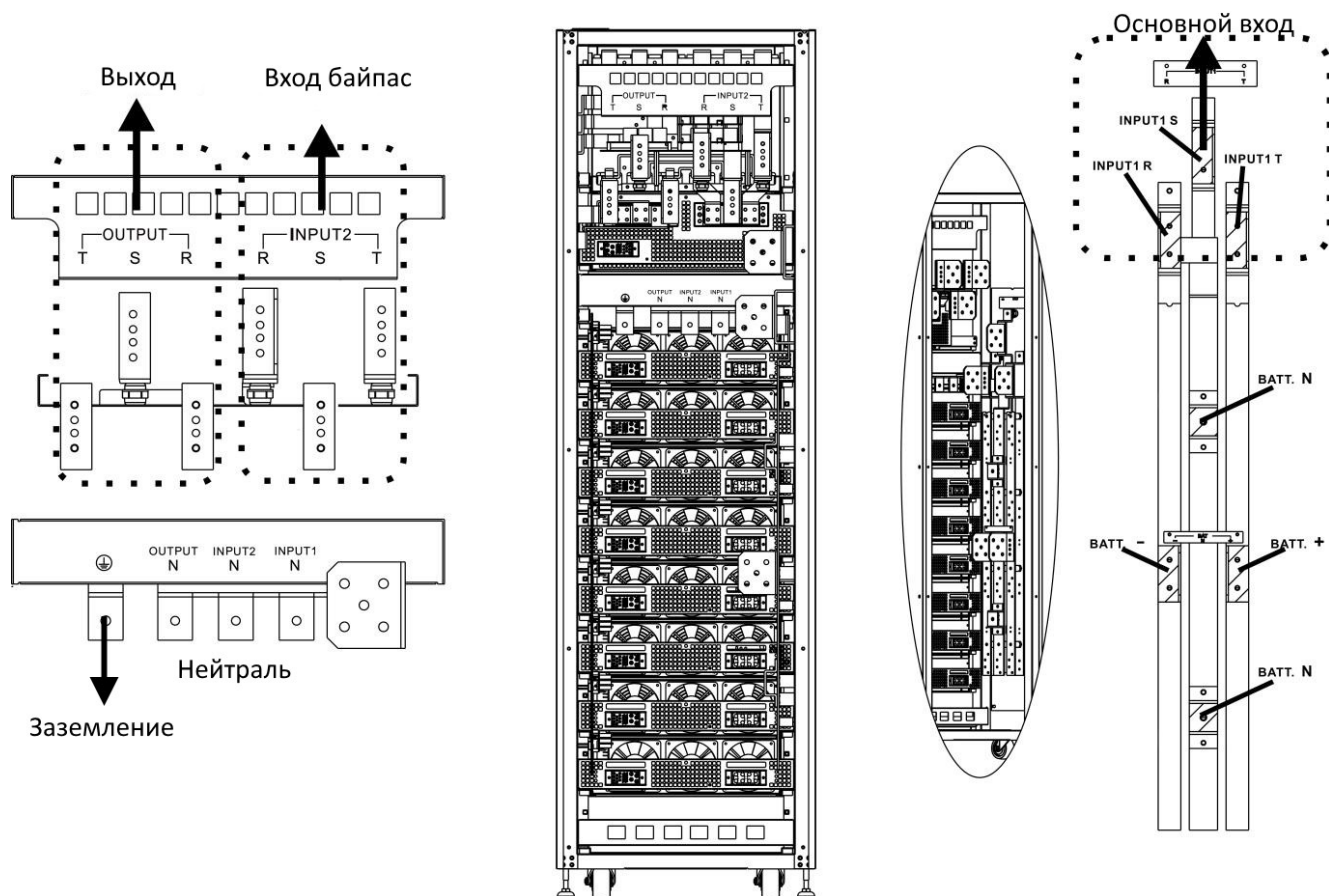
Рисунок 9. Шины подключения XM4 420.
